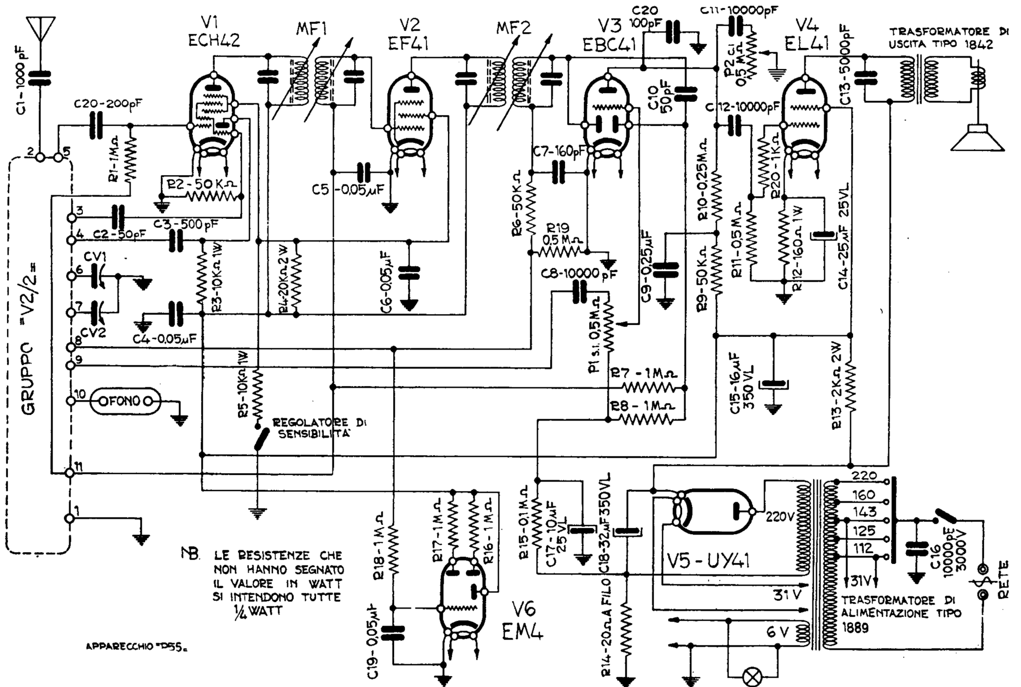
NOVA - Mod. P 55. Ricevitore con sintonia a permeabilità variabile, provvisto di gruppo AF mod. V 2/2. Media frequenza a 465 kc/s. Potenza indistorta di uscita 3,5 watt. Consumo 42 watt.
